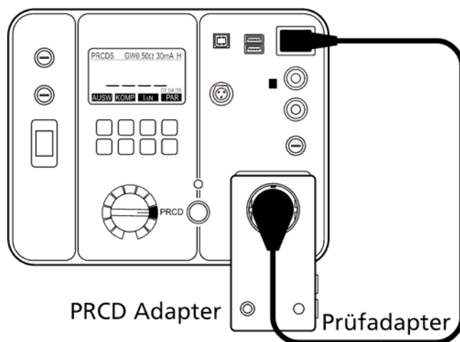
Abb. 36: Anschluss des PRCD Adapters für die Kompensation
