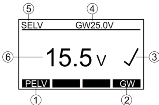
Abb. 45: Anzeige bei der SELV Prüfung (Beispiel)
