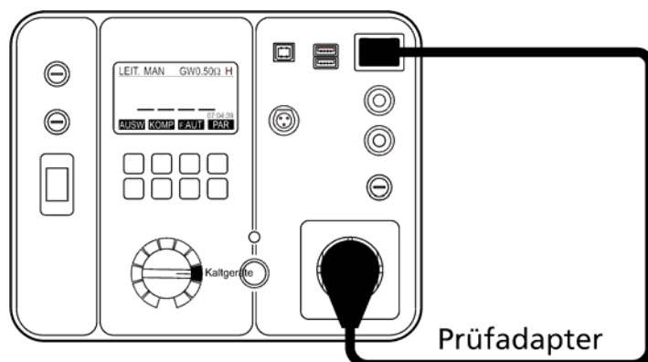
Abb. 33: Anschluss des Prüfadapters für die Kompensation
