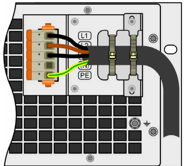
Bild 11 - Fertig montierte Zugentlastung
