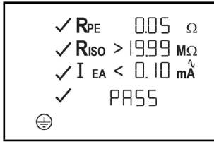
Zie fig. 3: Testen van apparaten van beschermklasse I (apparaten met aardegeleider en aanraakbare geleidende onderdelen die op de aardegeleider zijn aangesloten)
