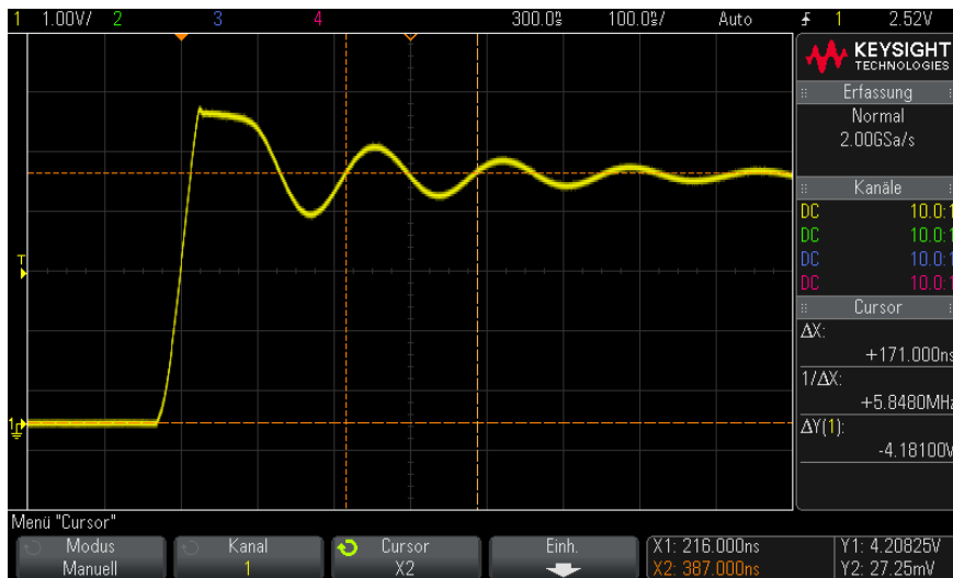
Abbildung 41 Cursor messen Überschwingfrequenz
