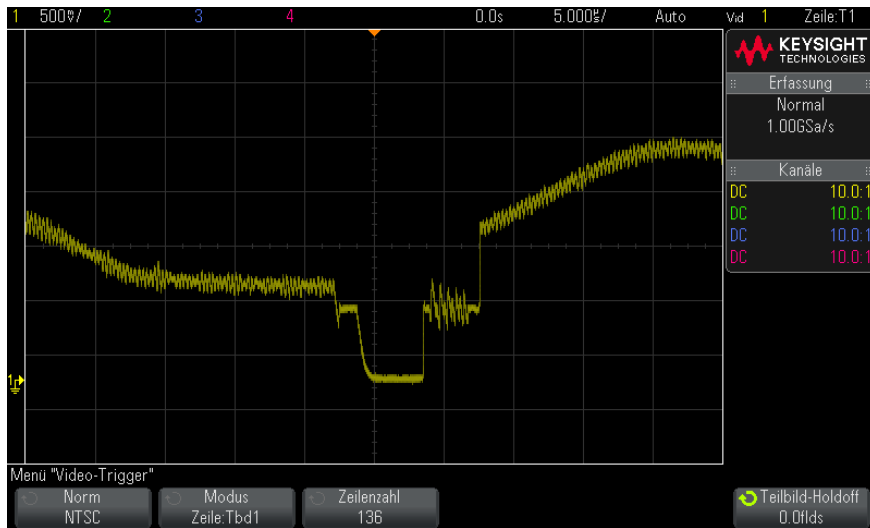
Abbildung 27 Beispiel: Triggerrung auf die Zeile 136
