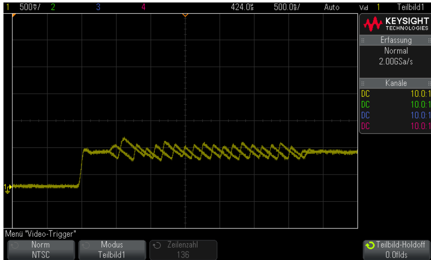
Abbildung 31 Abwechselnde Triggerrung auf die Farbteilbilder 1 und 3
