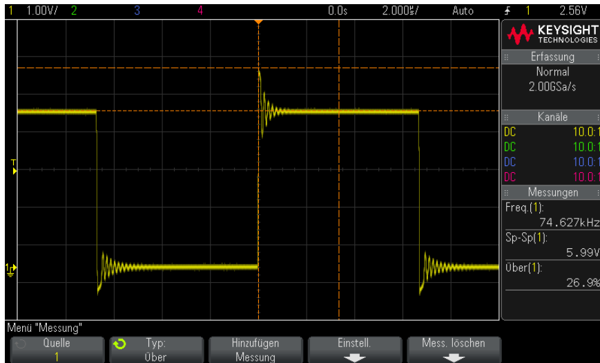
Abbildung 47 Automatische Messung des Überschwingers
