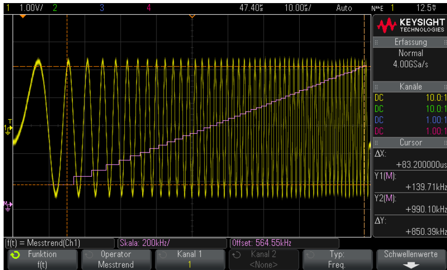
Abbildung 17 Beispiel für Messungstrend
