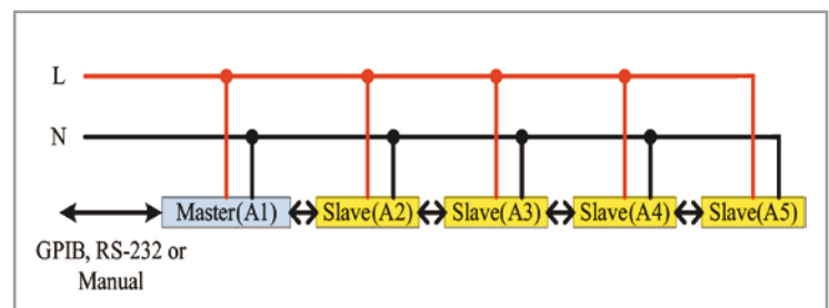
Abbildung 10: Parallelschaltung
