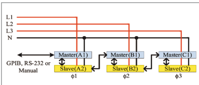
Abbildung 11: Paralleler/3-Phasen-Y-Anschluss
