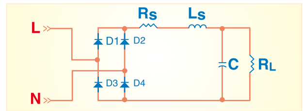
Abbildung 2: Typischer gleichgerichteter Schaltkreis
