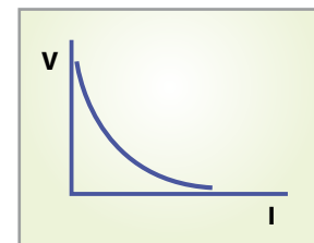
Konstante Leistung
