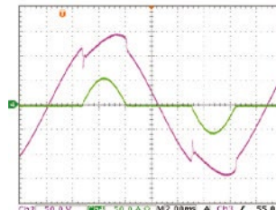
Abbildung 5: CC-Modus
