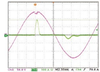
Abbildung 6: Einschaltstrommodus
