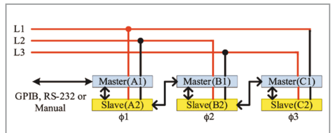
Abbildung 12: Parallele/3-Phasen-Dreieckschaltung
