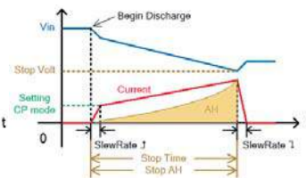
CP Mode
