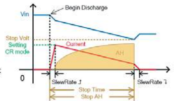
CR Mode
