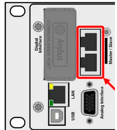
Bild 7 - Master-Slave-Busanschlüsse
