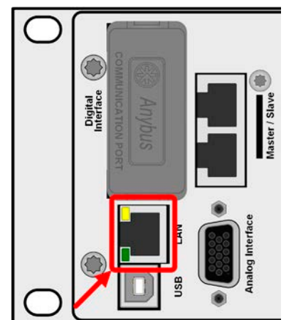
Bild 8 - LAN-Port
