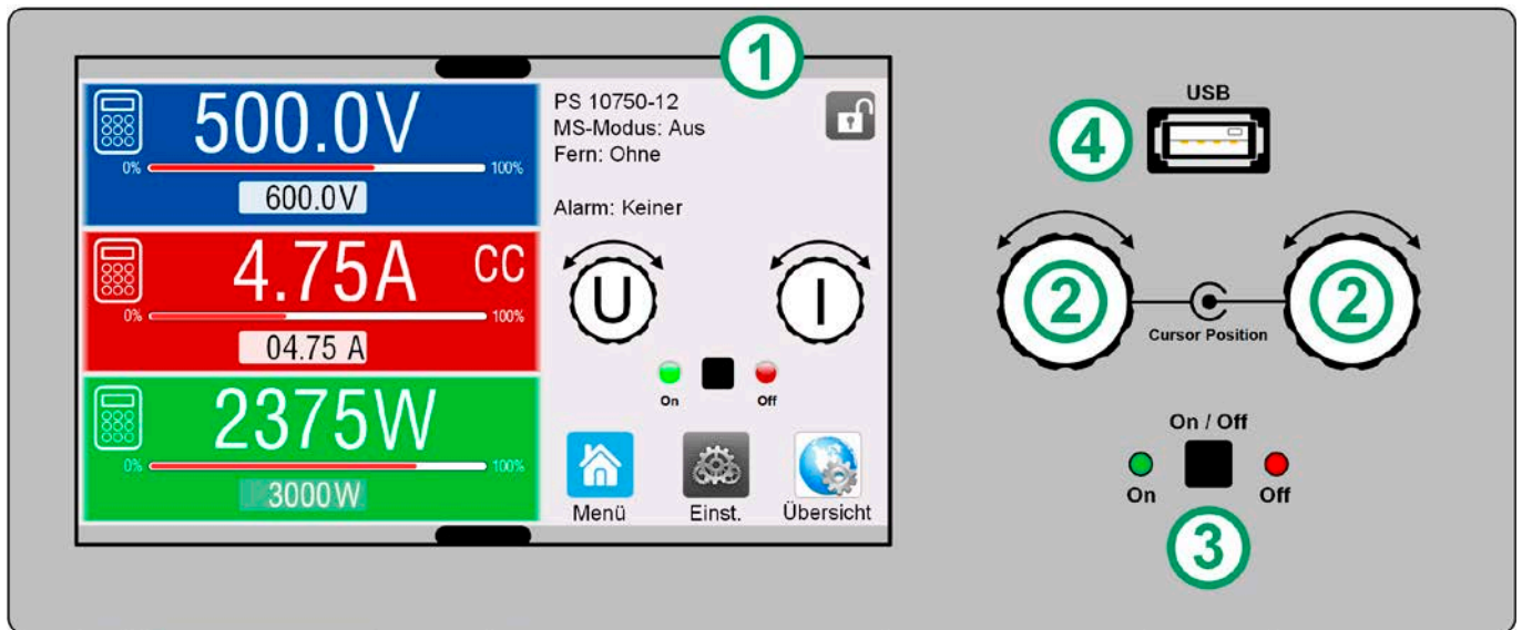
Bild 1 - Bedienfeld
