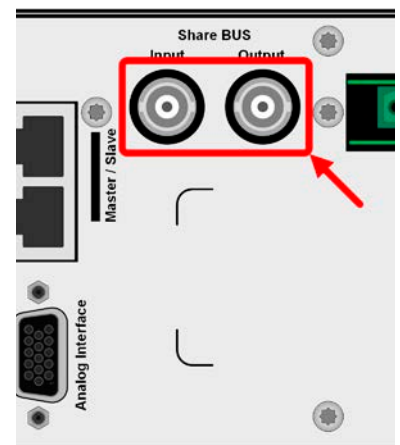
Bild 5 - Share-Bus
