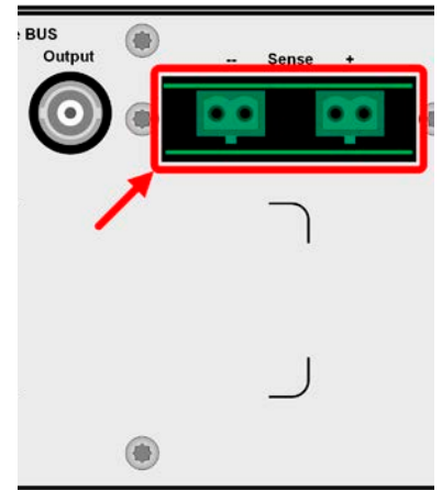
Bild 6 - Fernfühlungsanschlüsse
