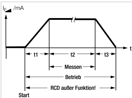
Unterdrückung der RCD-Auslösung bei pulsstromsensitiven RCD-Schutzschaltern
