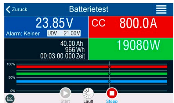
Bild 16 - Anzeigebispiel vom statischen Entladen
