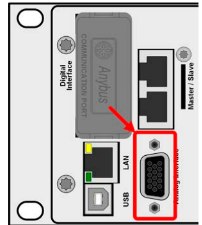
Bild 4 - Analogschnittstelle
