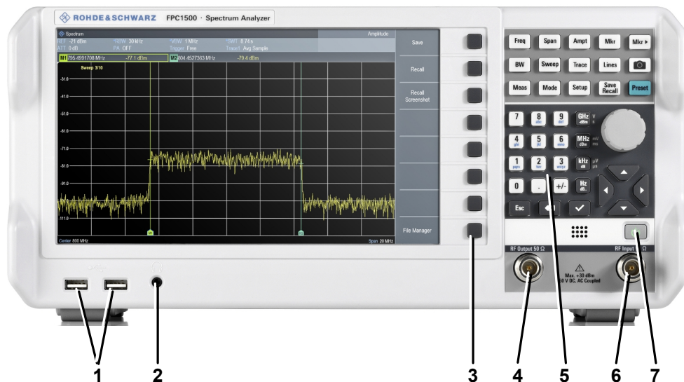
Bild 4-1: Frontplatte des R&S FPC
