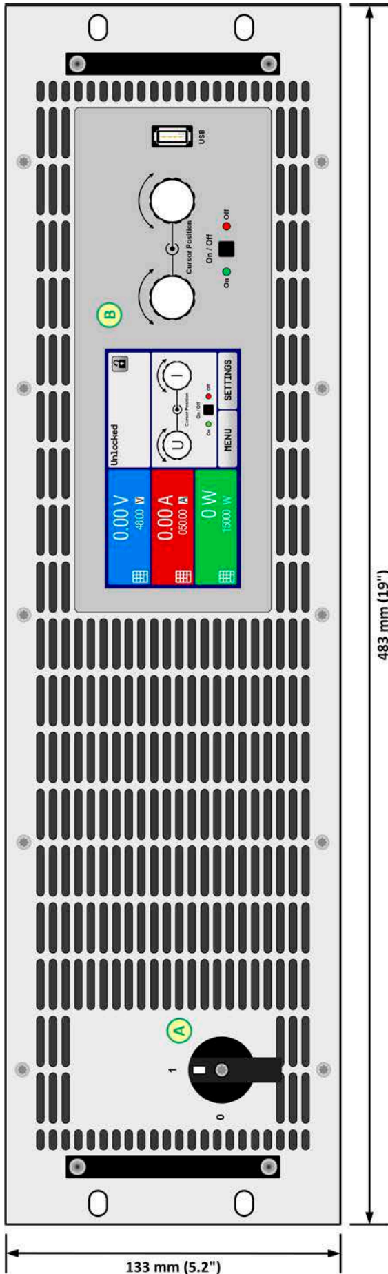
Bild 1 - Vorderseite (Standardausführung)
