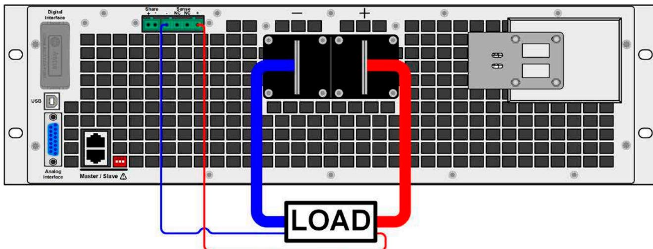
Bild 10 - Beispiel Fernfühlungsverdrahtung
