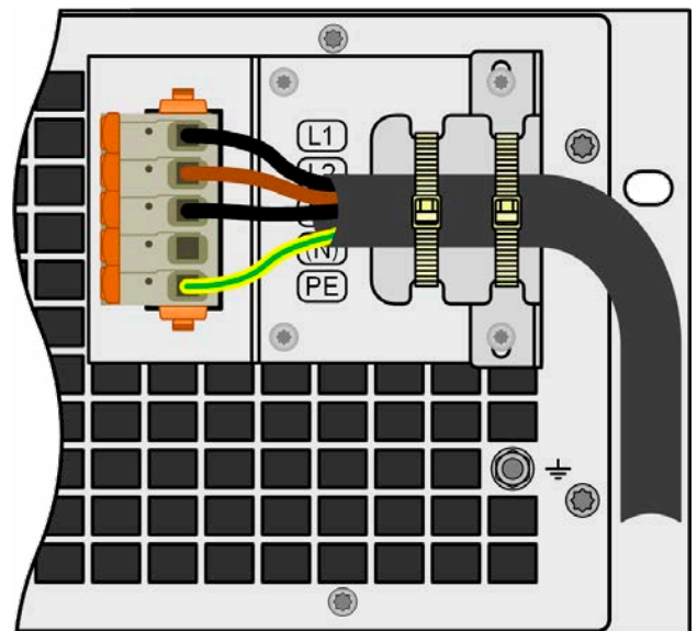
Bild 11 - Fertig montierte Zugentlastung
