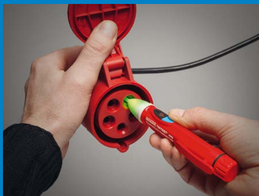
Drehfeldrichtungsprüfung an CEE-Kupplung mit TRITEST® easy
