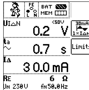
RCM-Prüfung
