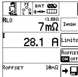
Niederohmmessung 25 A
