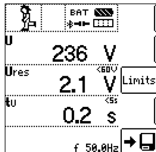
Restspannungsmessung
