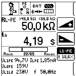
IMD-Prüfung
