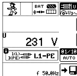
Spannungsmessung
