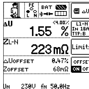
Spannungsfallmessung
