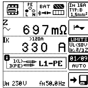
Schleifenwiderstandsmessung
