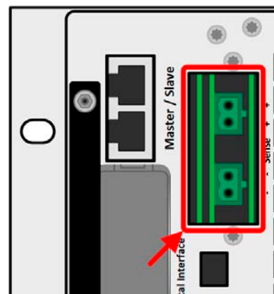
Bild 6 - Fernföhlungsanschlüsse
