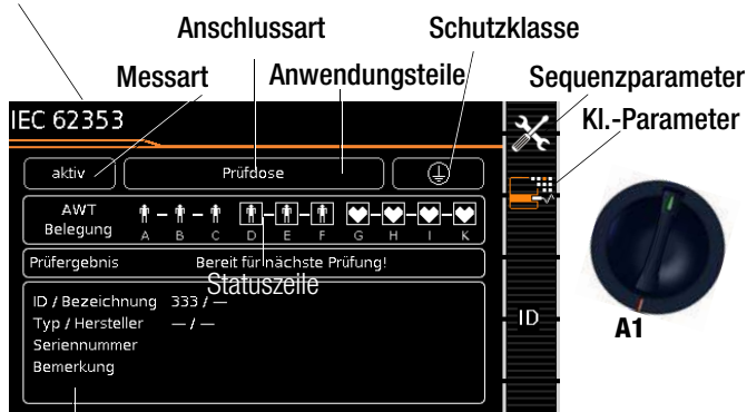
Detailansicht*
