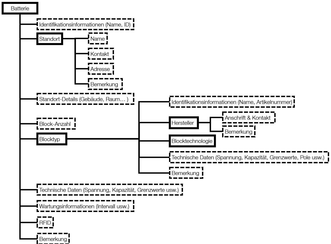
Bild 6: Datenbankstruktur: Einträge (——) und hinterlegbare Informationen (-----)
