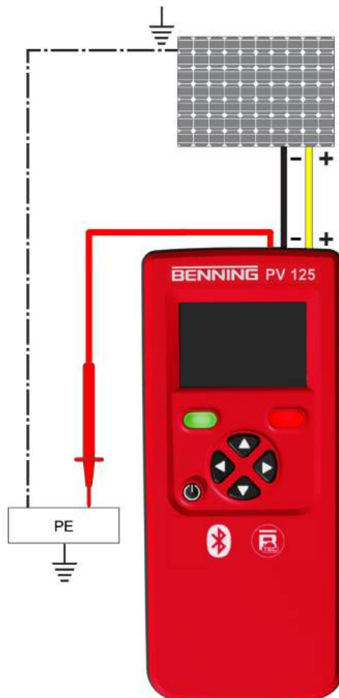
Abb. 10: Strang-Prüfung
