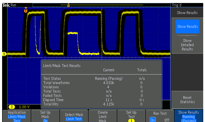
Grenzwerttest mit einer Maske, die mit einem idealen Signal generiert wurde und mit einem Echtzeit-Signal verglichen wurde. Ergebnisse, welche statistische Informationen über den Test anzeigen.
