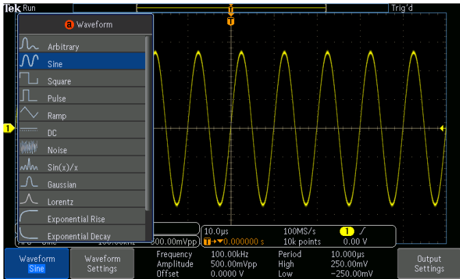
Signaltyp-Auswahl im integrierten AFG.
