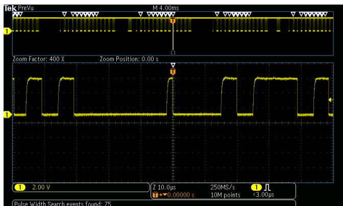
Suchen Schritt 2: Wave Inspector durchsucht automatisch die Aufzeichnung und markiert jedes Ereignis mit einem leeren, weißen Dreieck. Mit den Zurück- und Weiter-Schaltflächen gelangen Sie von einem Ereignis zum nächsten.
