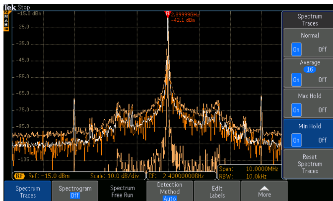
Anzeigetypen: Normal, Mittelwert, Max-Hold und Min-Hold
