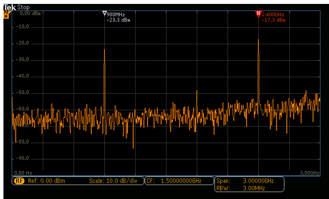
Spektralanzeige von gleichzeitig erfassten Zigbee-Bursts (900MHz) am Eingang und Bluetooth-Bursts (2.4GHz) am Ausgang eines Chips.
