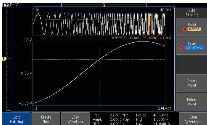
Arbiträr-/Funktionsgenerator-Editor mit Anzeige des Punkt-für-Punkt-Editors.
