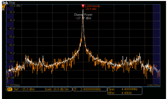
Automatische Kanalleistungsmessung
