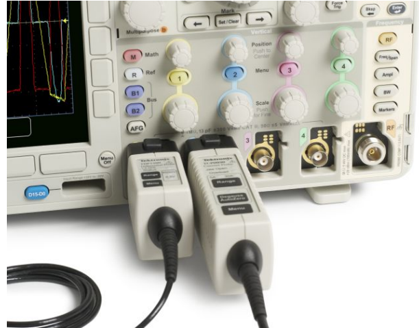
Die TekVPI-Tastkopfschnittstelle vereinfacht den Anschluss der Tastköpfe an das Oszilloskop.
