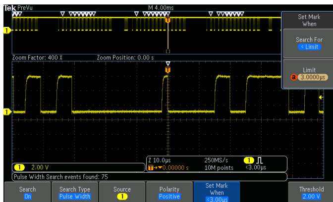
Suchen Schritt 1: Definieren Sie, wonach gesucht werden soll.
