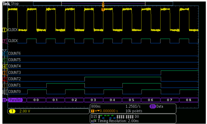
Das MDO3000 mit Option MDO3MSO bietet 16 integrierte Digitalkanäle für die Anzeige und Analyse von zeitkorrelierten analogen und digitalen Signalen.
