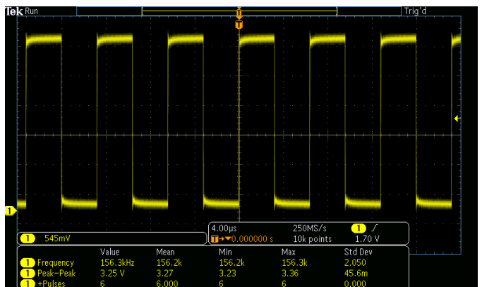
Automatische Messwertanzeigen ermöglichen wiederholbare, statistische Ansichten von Signaleigenschaften.
