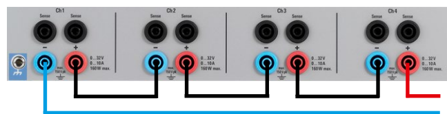
Serieller Betrieb – max. 128 V
