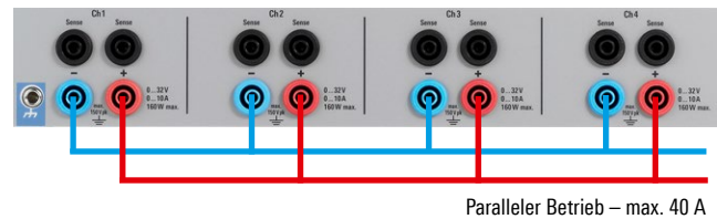
Paralleler Betrieb – max. 40 A
