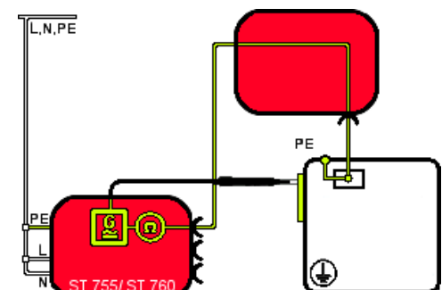
Stromlaufplan
