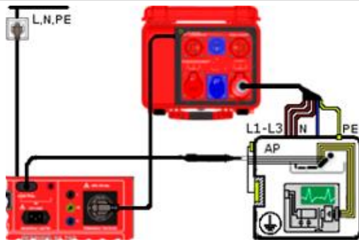
Anschlusschema
