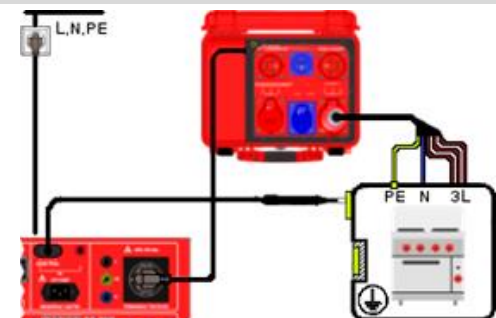
Anschlusschema
