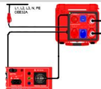
Anschlusschema
