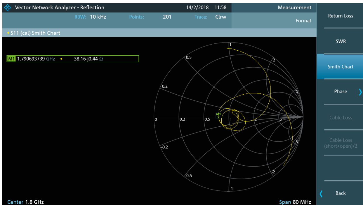
R&S®FPC1500: Smith-Diagramm mit R&S®FPC-K42 Option
