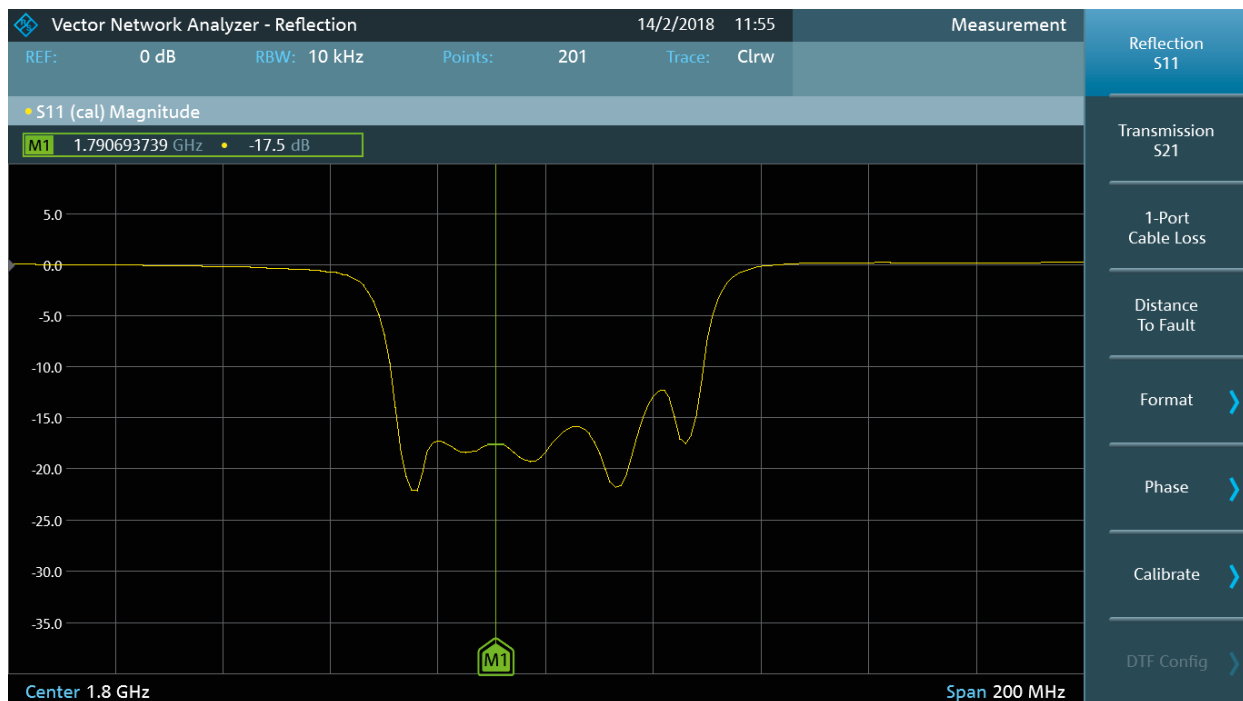
R&S®FPC1500: S_{11} -Betragsmessung mit der R&S®FPC-K42 Option
