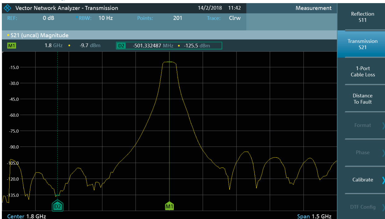
R&S®FPC1500: skalare S_{21} -Übertragungsmessung mit der R&S®FPC-K42 Option
