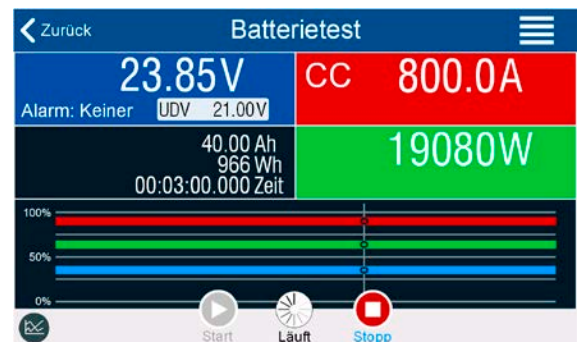
Bild 17 - Anzeigebispiel vom statischen Entladen
