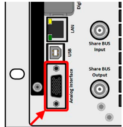
Bild 4 - Anlogschnittstelle
