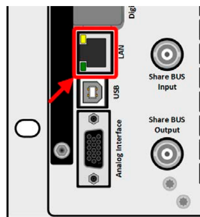
Bild 8 - LAN-Port
