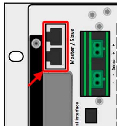
Bild 7 - Master-Slave-Busanschlüsse
