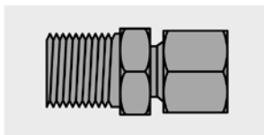
Anschluß: Winkelstück Außengewinde: M16x1,5
