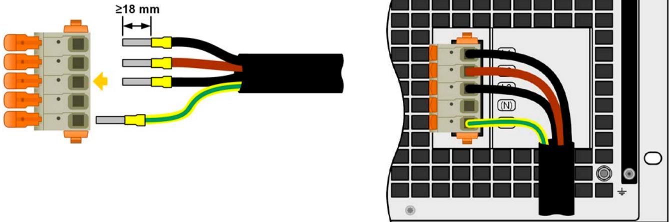
Bild 10 - Beispiel für ein Netzanschlußkabel mit 4 Adern (nicht im Lieferumfang enthalten)
