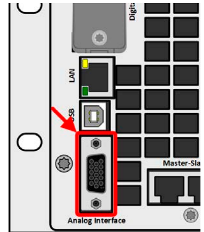
Bild 4 - Anologschnittstelle
