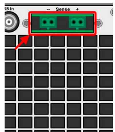
Bild 6 - Fernfühlungsanschlüsse
