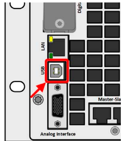
Bild 2 - USB-Anschluß
