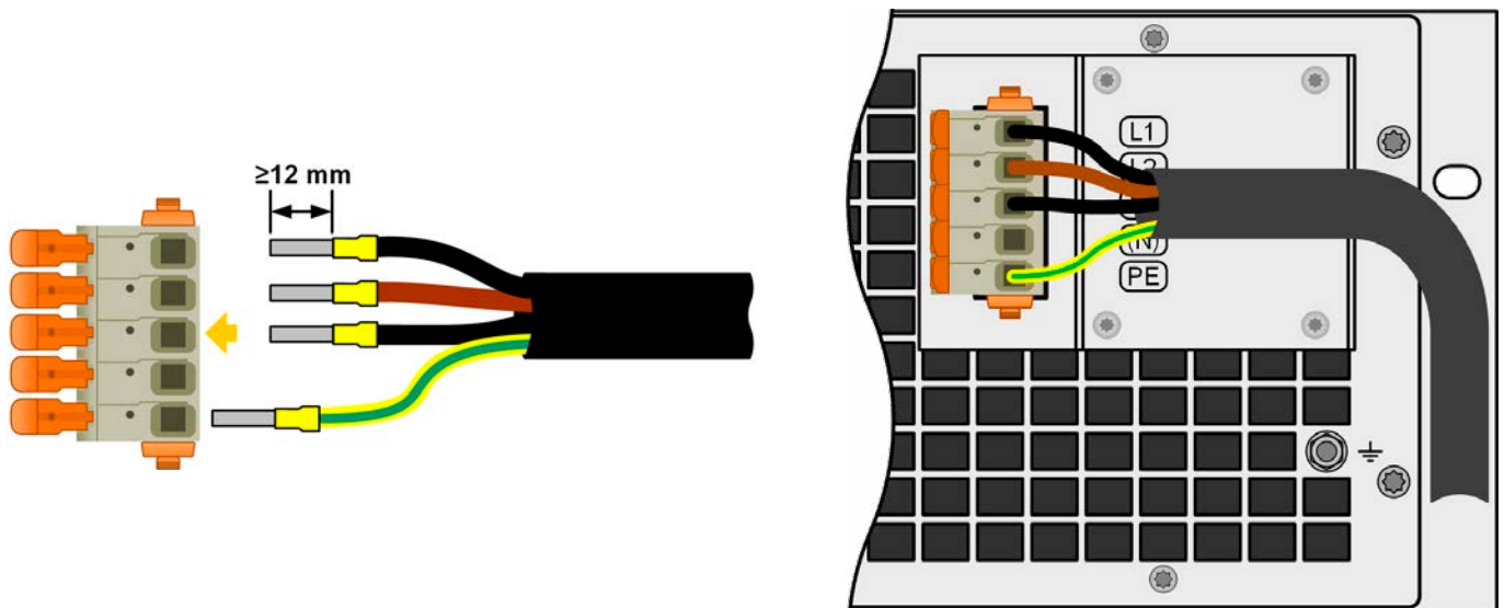
Bild 10 - Beispiel für ein Netzanschlußkabel mit 4 Adern (nicht im Lieferumfang enthalten)
