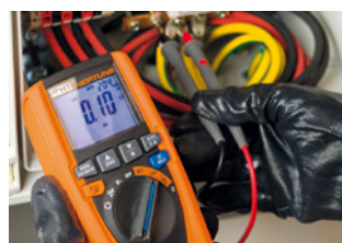
Durchgangsprüfung von Schutzleitern.
