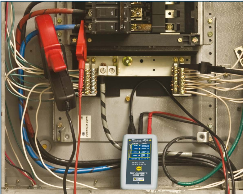
Überwachung von Strom und Spannung in einem Lastverteilungszentrum mit einem L562
