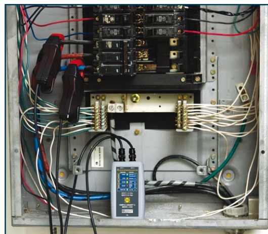
Stromaufzeichnung an 2 Außenleitern mit L102.
